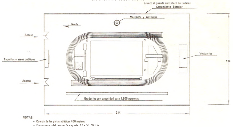
ESQUEMA DE LAS PISTAS DE ATLETISMO, CON CAMPO DE DEPORTES A REALIZAR POR EL ILMO. AYUNTAMIENTO DE AYAMONTE
